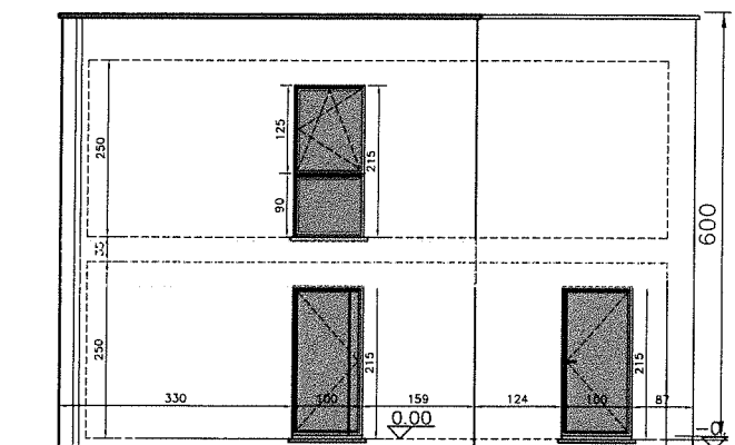
Achtergevel
