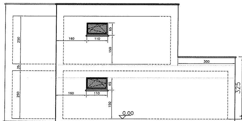
Zijgevel rechts
