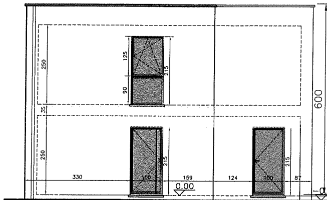
Voorgevel
