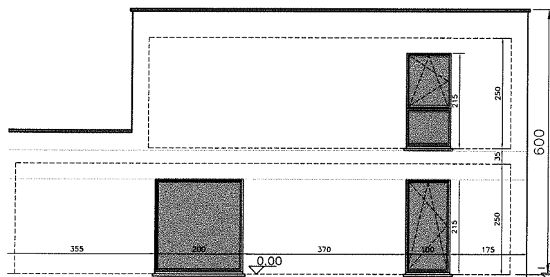
Zijgevel links
